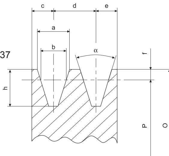
Pulley dimentions • Keilriemenscheibeabmessungen • Dimensions poulie • Dimensiones polea
