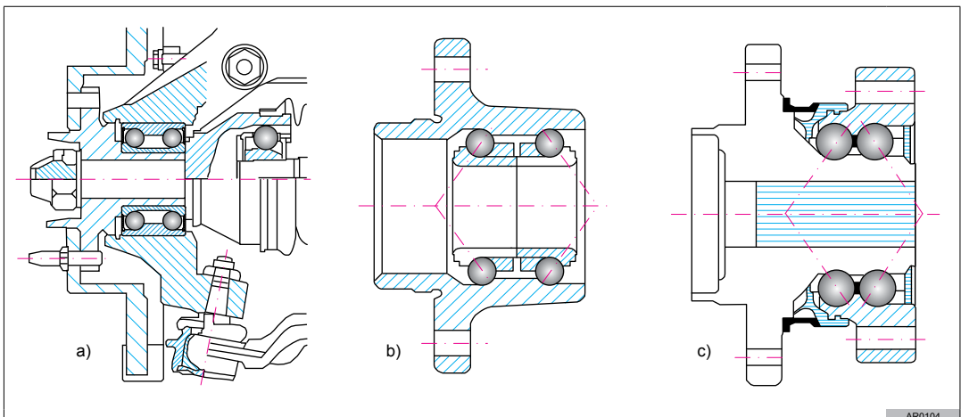
Rys.4 Zespólna piasta:
